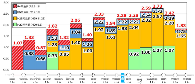
▲有明海沿岸道路の断面交通量の変化（初開通直後(H20.6)から現況(R4.11諸富IC開通後)までの変化)
